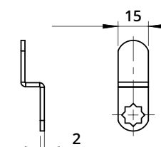
Leva piegata vedi pag. 196-197 For bent cam plate refer to page 196-197
