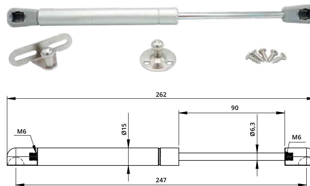
FORZE DISPONIBILI - AVAILABLE FORCES
