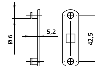
Leva con perni ad asta vedi pag. 197 For cam plate with lock bar pins refer to page 197
